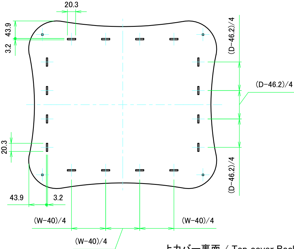
上カバー裏面 / Top cover Backside
