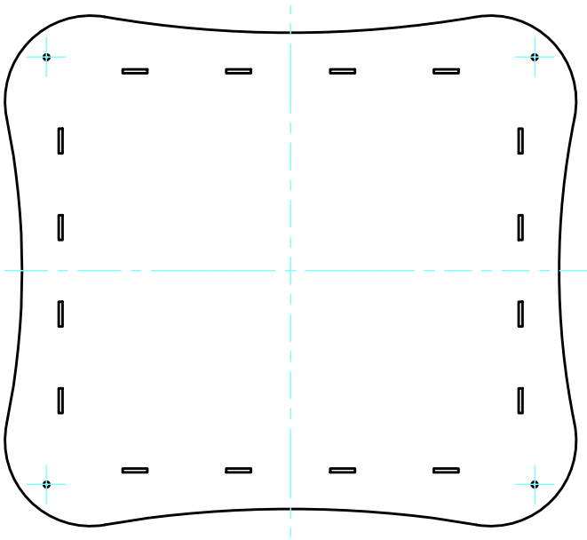
下カバー表面 / Bottom cover Frontside
