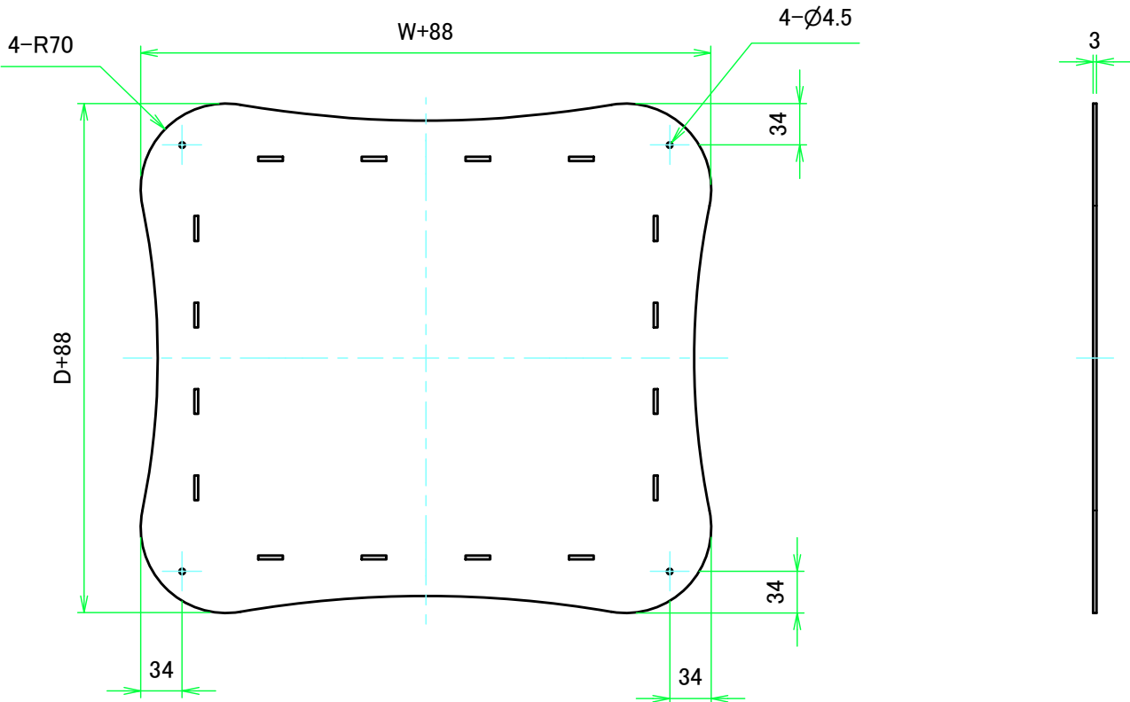
上カバー表面 / Top cover Frontside
